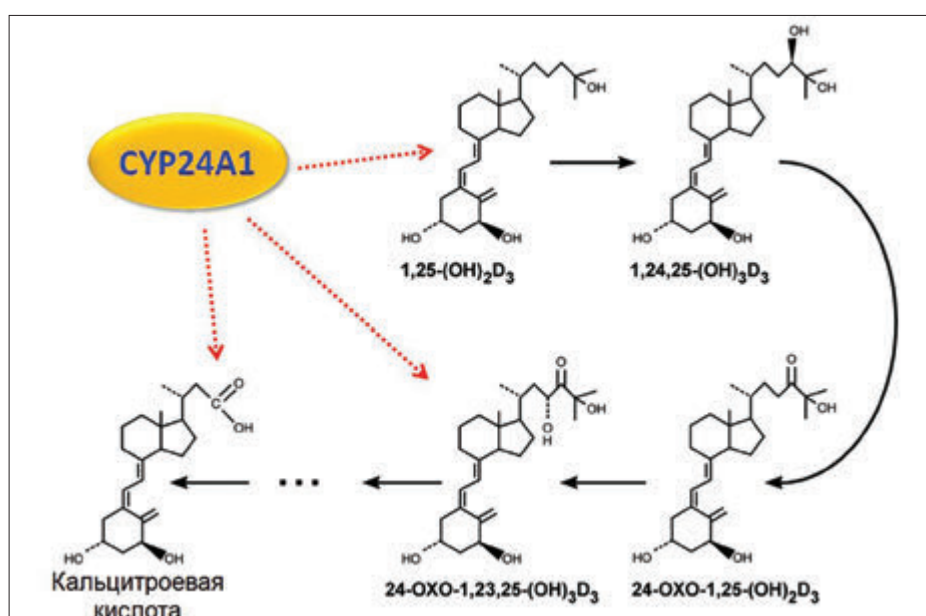
Рис. 3. Дegrадация 1,25(OH) 2 D 3
