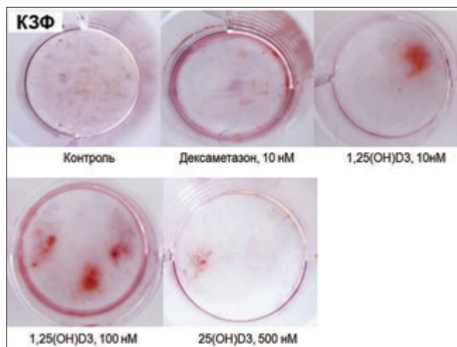
Рис. 6. Биоминерализация клеток зубного фолликула (К3Ф) при воздействии метаболитов витамина \text{D}_3 . Окрашивание клеток, в которых был стимулирован остеогенез, производилось ализариновым красным. Проведено сравнение с дексаметазоном (глюкокортикостероид, наиболее часто используемый для индукции остеогенеза)
